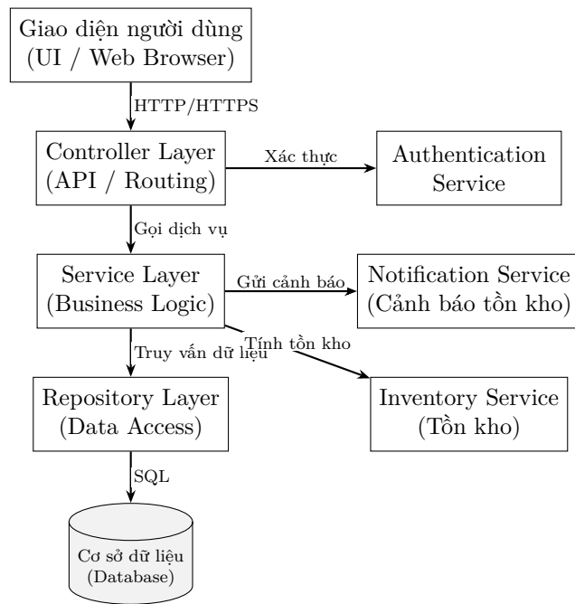
Figure 1: Component Diagram – Kiến trúc thành phần hệ thống quản lý kho hàng
